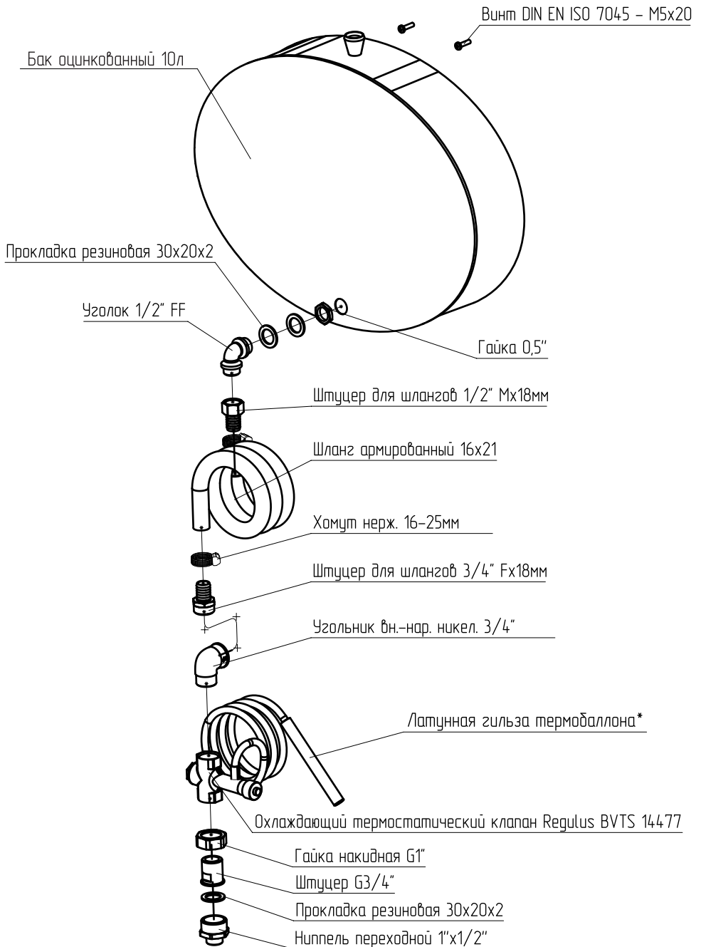
Рис.1 Схема сборки системы охлаждения топливопровода.
