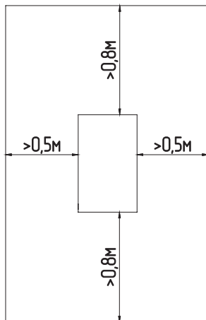
Рис.4 Схема размещения котла в помещении
