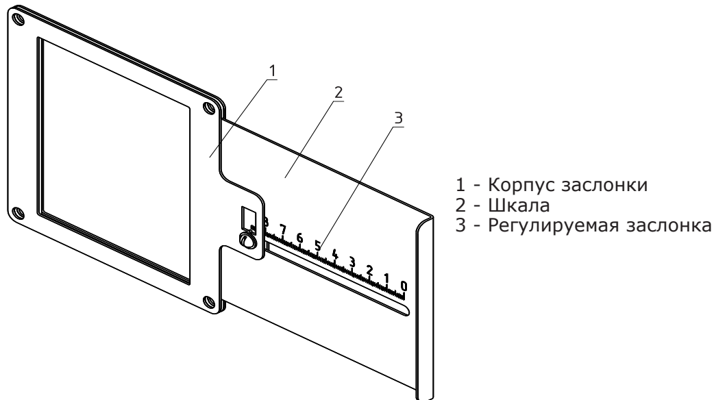
Рис.12 Заслонка вентилятора
