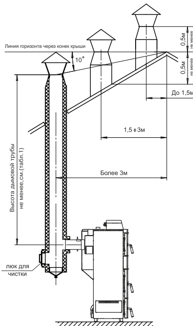
Рис.8 Варианты установки дымовой трубы
