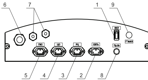
Рис.6 Расположение органов управления на задней панели пульта
