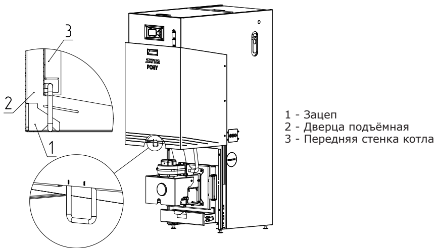
Рис.2 Зацеп двери
